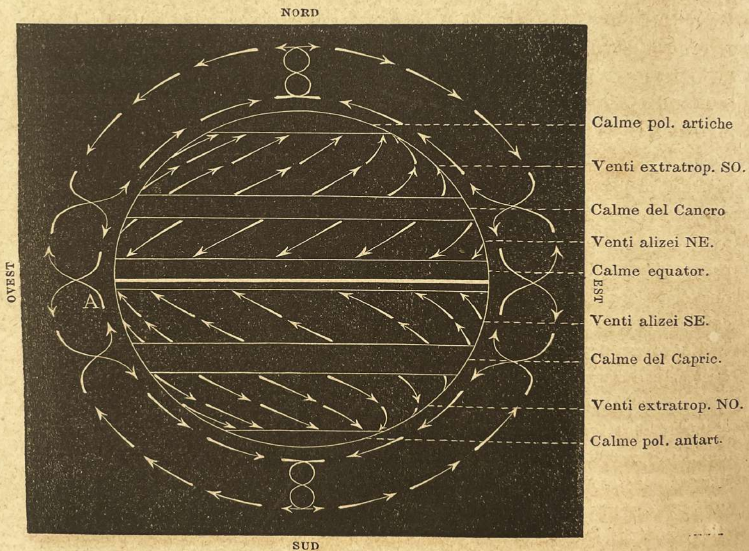
Fig. 2. Circolazione atmosferica secondo il sistema di Maury.
