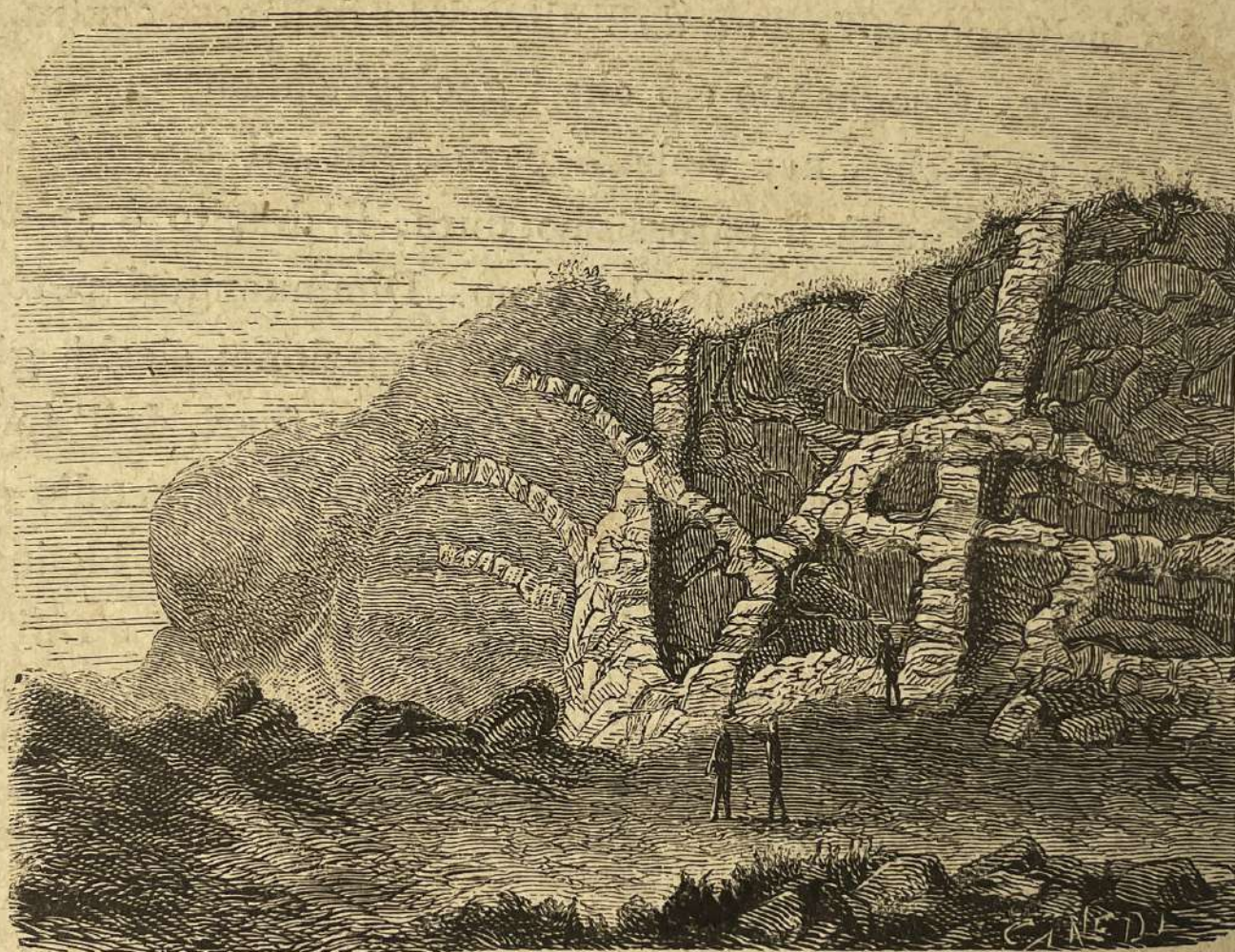
Flg. 61. Dicchi del monte Somma veduti dall'Atrio del Cavallo.
