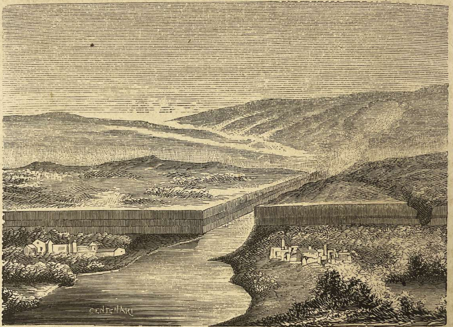
Fig. 14. Veduta del Niagara.
