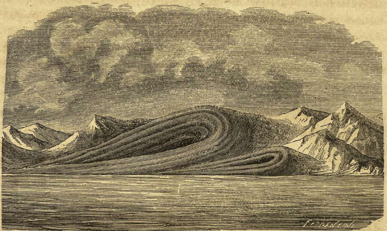
Fig. 83. Cratere dell'Ottmann Boss.
